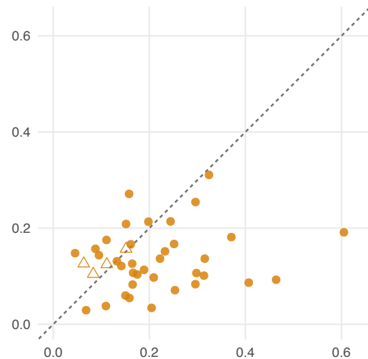
D Qwen3.6-Plus
