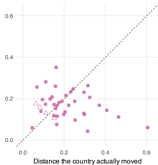
D Qwen3.6-Plus
