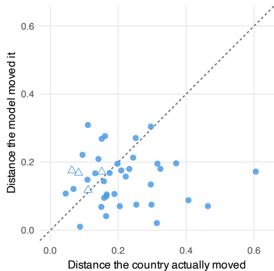
C GPT-5.5
